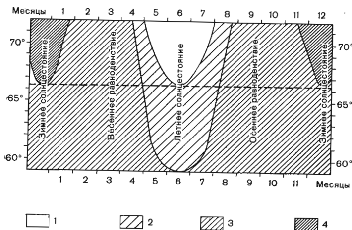
Рис. 3. Периоды солнечного освещения между 72 и 59° с. ш.:
