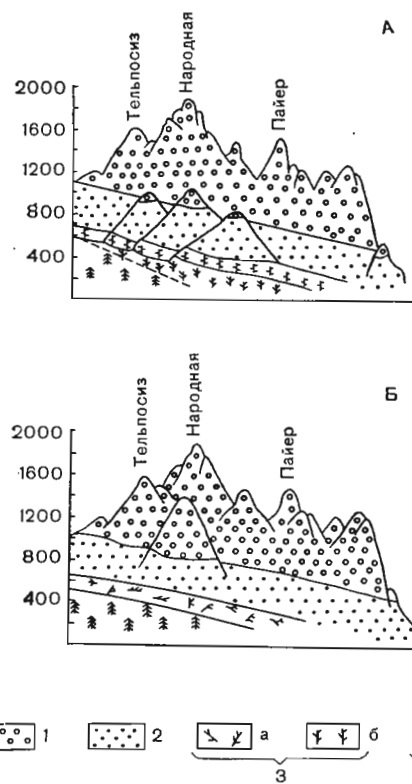
Рис. 50. Распределение высотных зон на восточном (А) и западном (Б) склоне Урала (по П. Л. Горчаковскому):
