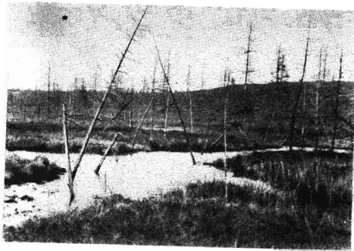
Рис. 20. Термокарстовое озеро в пересечении ледяных жил-клиньев (фото Л. Ведерникова)
