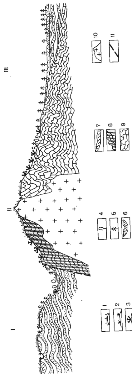
Рис. 37. Ландшафтный профиль Алазейской провинции (составил автор):
