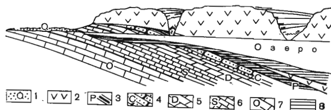
Рис. 46. Строение впадины оз. Лама (составил автор):
