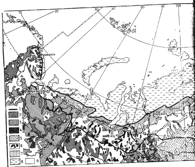
Рис. 23. Распределение редколесий и реди
