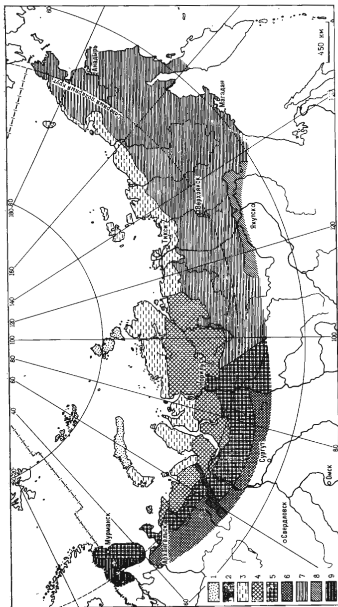
Рис. 24. Типы болот (по Н. Я. Кацу)
